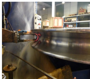
Kabelschijf met spoel
